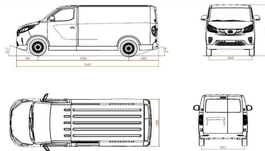
MAXUS eDELIVER 3 L2
